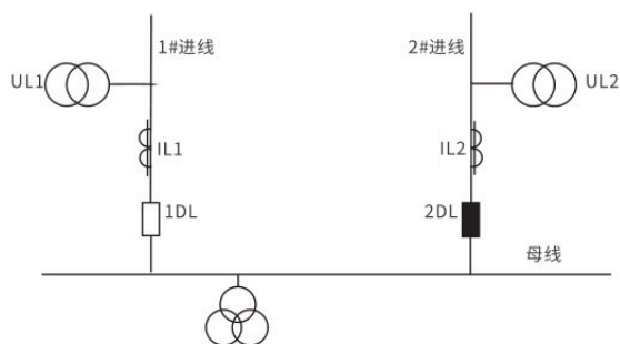
图1 两进线回路之间的快速切换主接线
